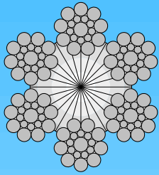
6x19S-FC Seale
