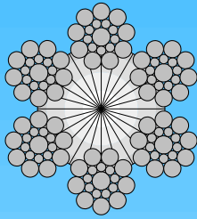
6x19F-SFC Filler
