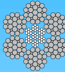
6x25F-IWRC Filler
