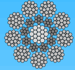
9x25F-PWRC Filler
