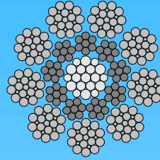
9x21F-PWRC Filler
