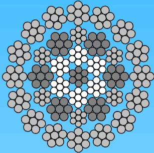
35(W)x7 Rotex-Plus
